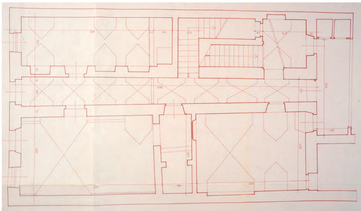
План основе зграде апотеке „Код златног орла“ у Петроварадину
